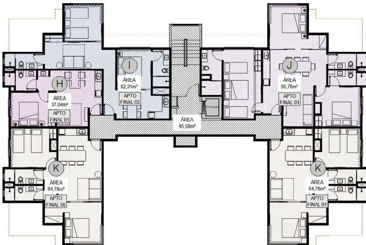
Figura 3 - BLOCO A1, A2, A3 e A4 - COBERTURA.
