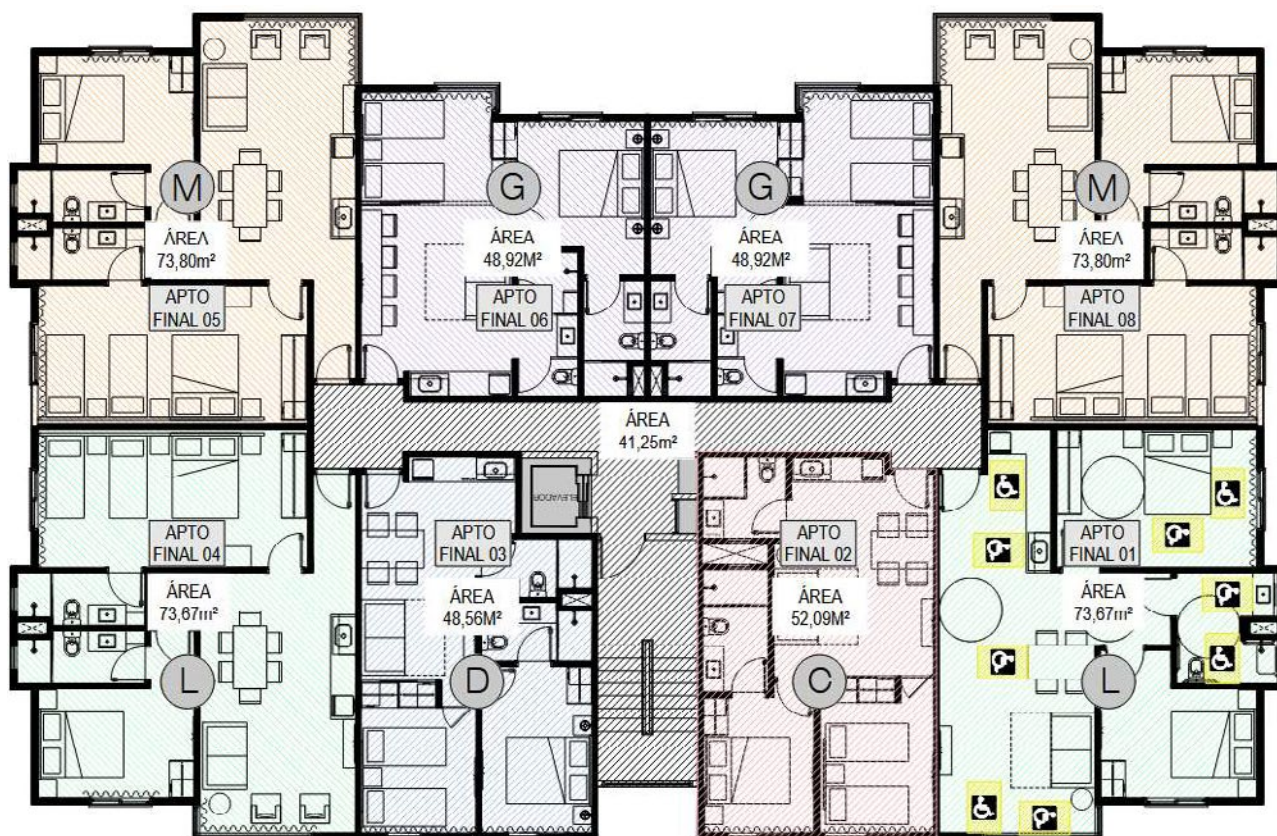
Figura 5 - BLOCO B5, B6, B7, B8, B9 e B10 – 1º e 2º PAVIMENTO.
