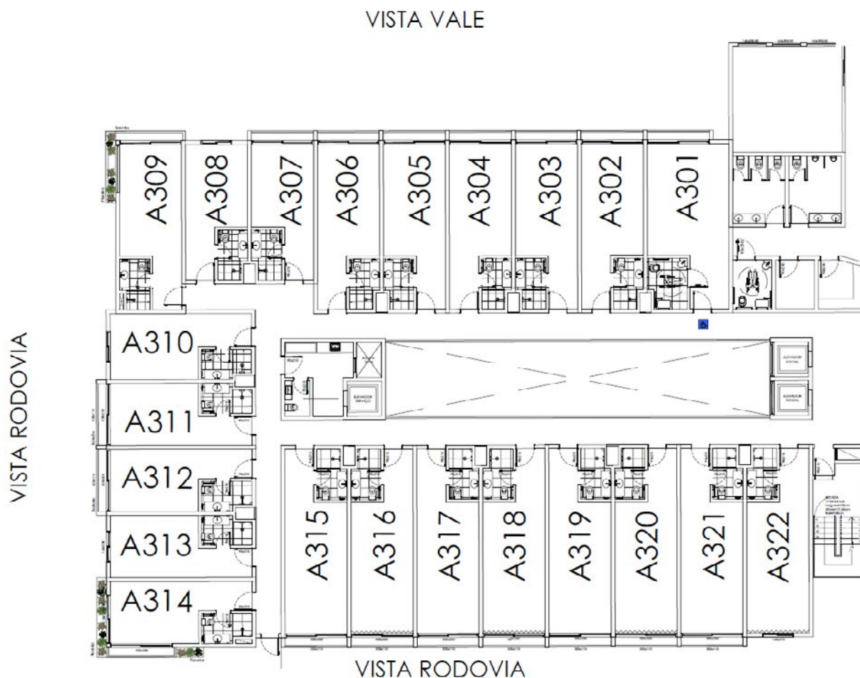
BLOCO A - SUB 1/ TÉRREO / 1º PAV.
